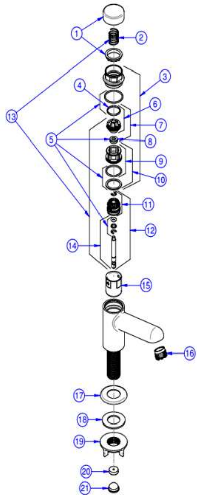
Aireador antivandalismo
