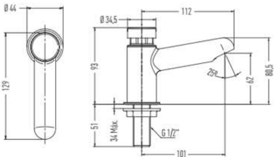
DIMENSIONAL (medidas en mm)
