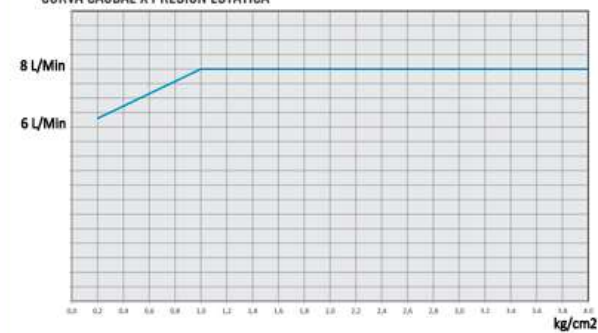
CURVA CAUDAL X PRESIÓN ESTÁTICA
