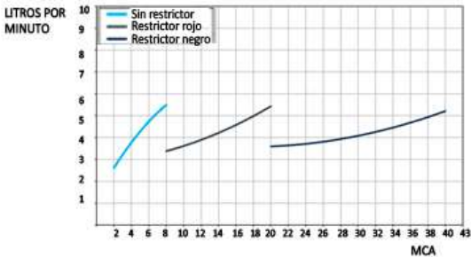
CURVA DE CAUDAL
